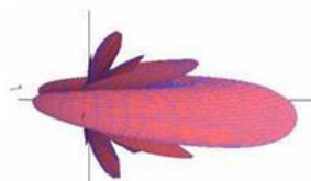
Antennen- Richtcharakteristik
